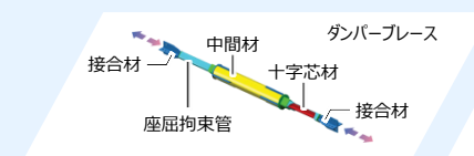
“制振装置（TMD）”により 地震対策、性能UP
